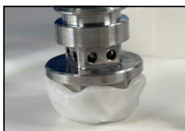
Renfort mécanique en Re-FORM sur une pièce fragile.
